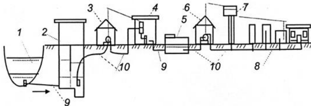
Рис. 1. Общая схема водоснабжения населенного пункта:
