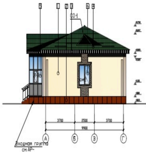
Фасад по осям А-Г М 1:100
