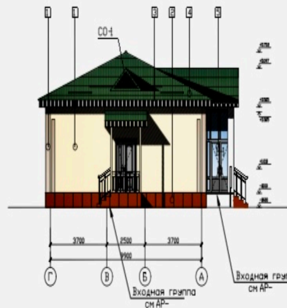
Фасад по осям Г-А М 1:100
